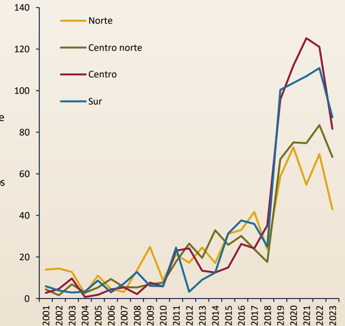
Número de días acumulados por región en el año clasificados como ondas de calor de enero de 2001 a junio de 2023
